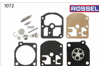
Código: 27645 Reparo carb. St.FS-160/220/280 + kit agulha mod.zama
