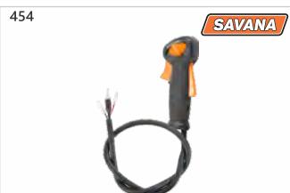
Código: 25494 Empunhadura aceleração 43cc/S430 22mm completa
