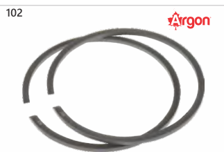
Código: 16878 Anel compressão St.260 44,7x1,2mm
