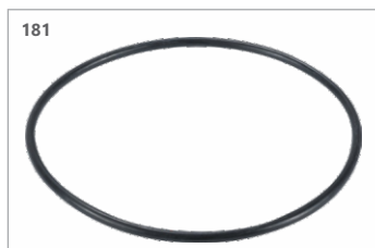
Cód.: 07768 Oring 72,69x2,62 K3xx
