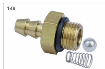
Cód.: 28581 Niple sucção (aspiração de detergente) K3-K4 hx...9.303-344.0
