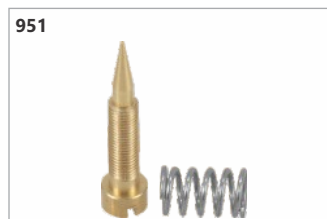
Código: 21654 Parafuso ajuste ar 15hp Yamaha (com mola)
