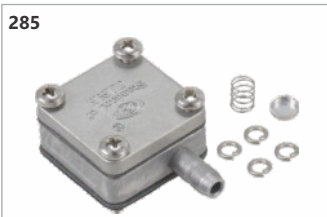
Código: 22607 Bomba combustível cpl. 4,0hp Yamaha
