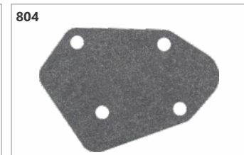
Código: 19392 Junta superior carburador 40hp Yamaha
