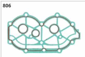
Código: 16938 Junta tampa cabeçote 25hp Yamaha
