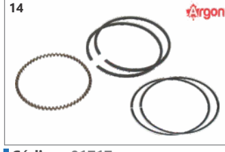
Código: 01717 Anel compr. 60mm std. (jogo) 4,0hp
