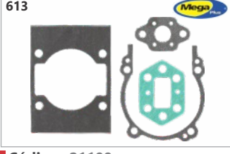
Código: 21109 Jogo juntas Husq. 236 / 143RII (Mega Plus)
