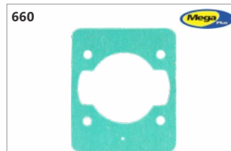
Código: 02675 Junta cilindro Husq. 142R (Mega Plus)
