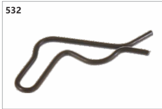
Código: 00105 Grampo elástico partida simples St. 038/051/066/076/350/650/651 /660/760/P835/840
