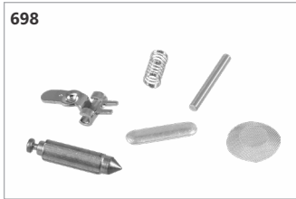
Código: 02508 Kit agulha Zama Echo 2300
