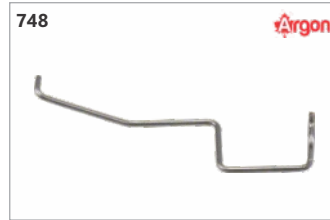
Código: 23942 Mola gatilho acelerador motosserras 45/52/58cc (Argon)
